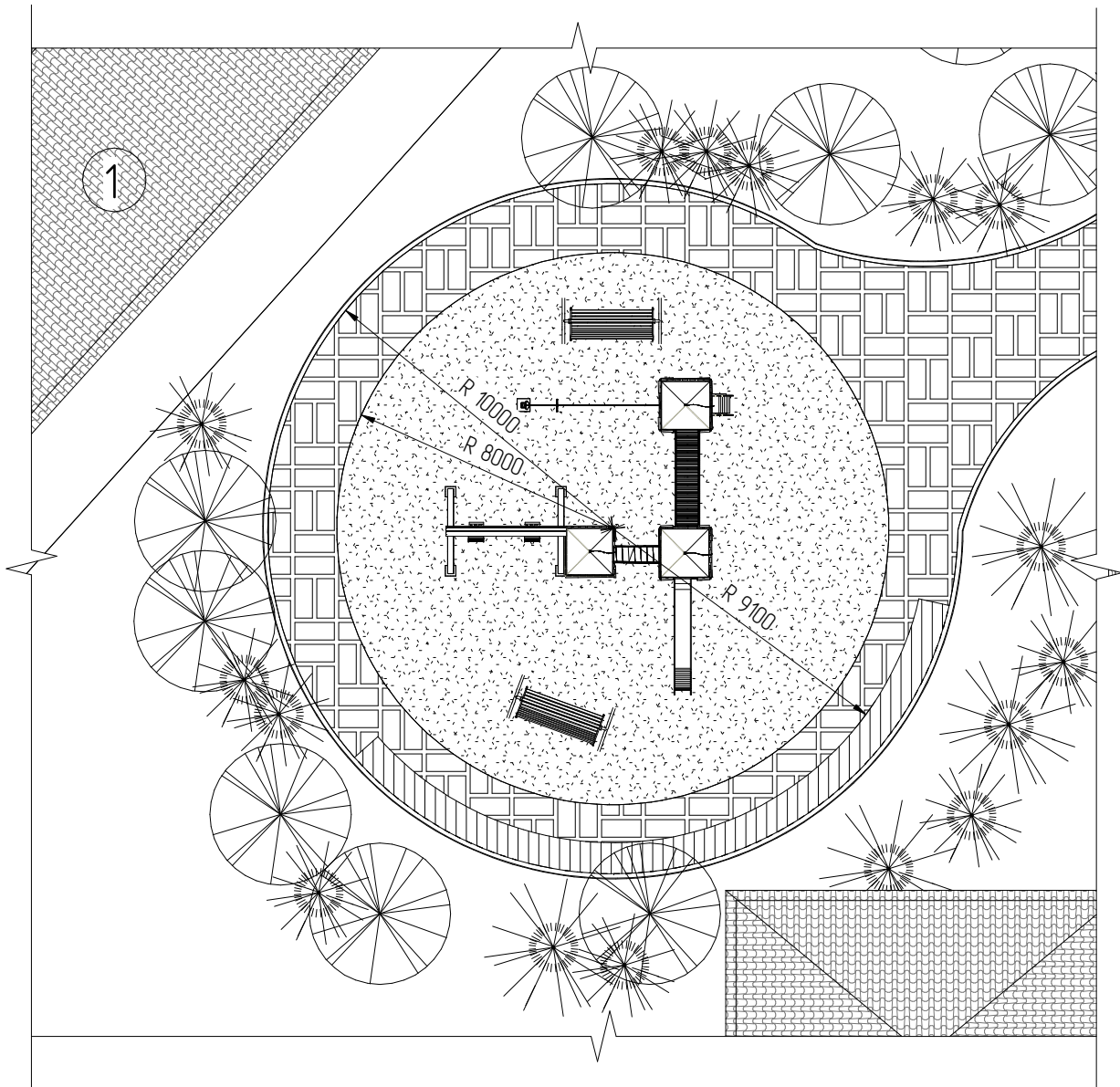
Площадка №3 (ситуационный план)
